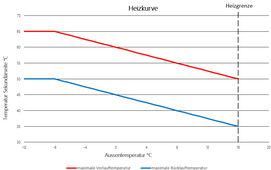
Abbildung 2: Heizkurve
